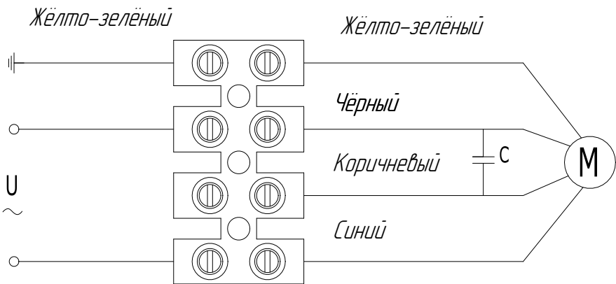
СХЕМА ПОДКЛЮЧЕНИЯ
